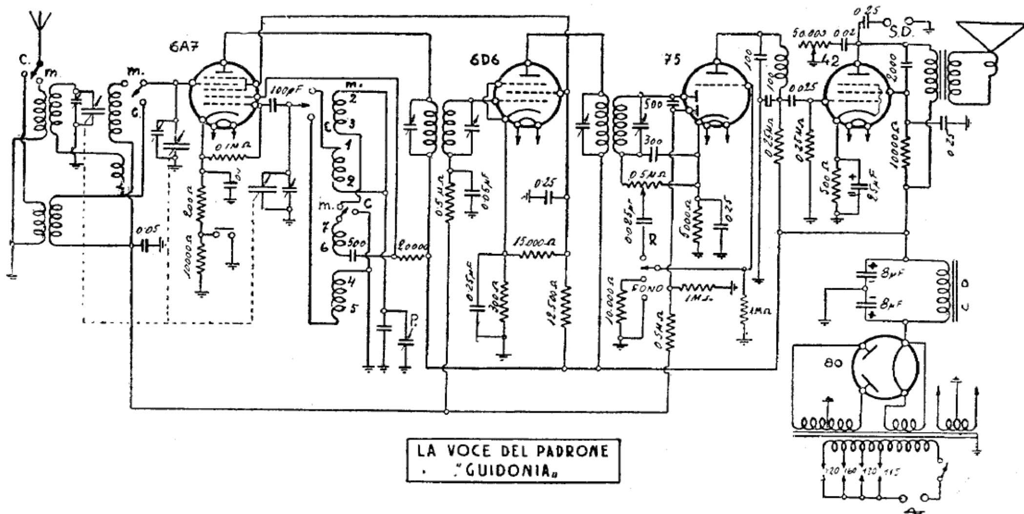
LA VOCE DEL PADRONE. — Mod. « Guidonia ». - Produzione 1937. - Media frequenza: 175 kHz.
